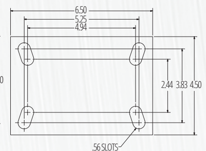
OPTIONAL 42ST/42RT TOP PLATE
