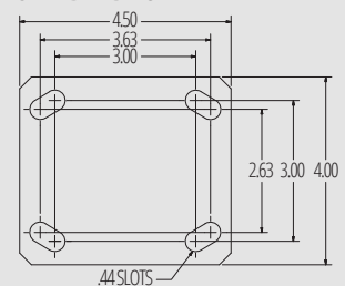
OPTIONAL 42ST/42RT TOP PLATE
