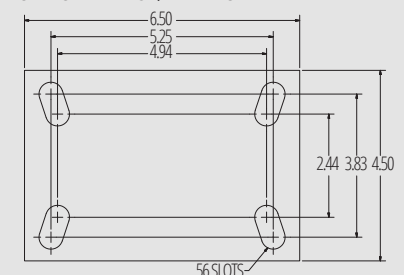
OPTIONAL 42ST/42RT TOP PLATE
